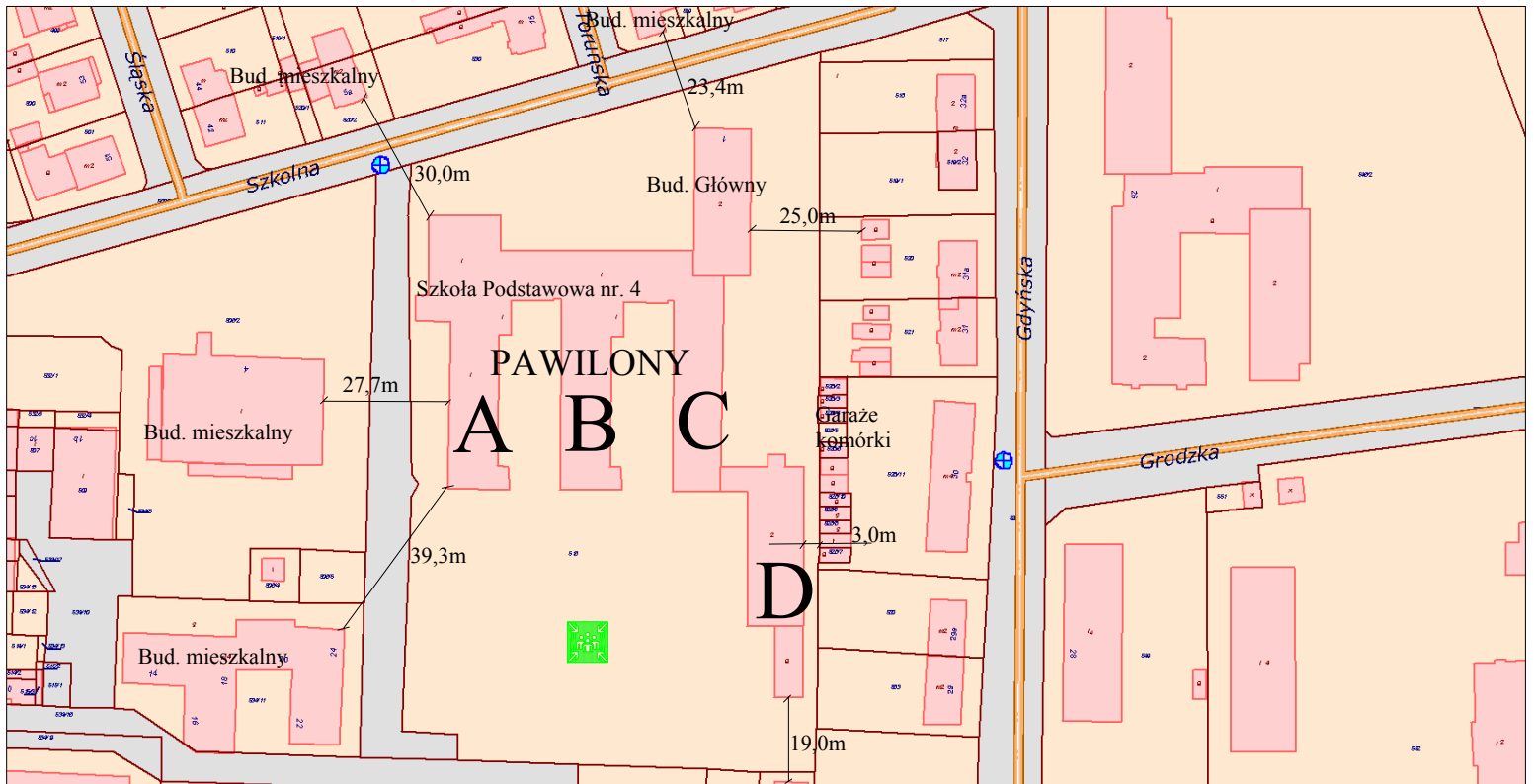
Rys nr 10 Załącznik do IBP. Oznaczenie odległości od innych obiektów i oznaczenie hydrantów zewnętrznych
